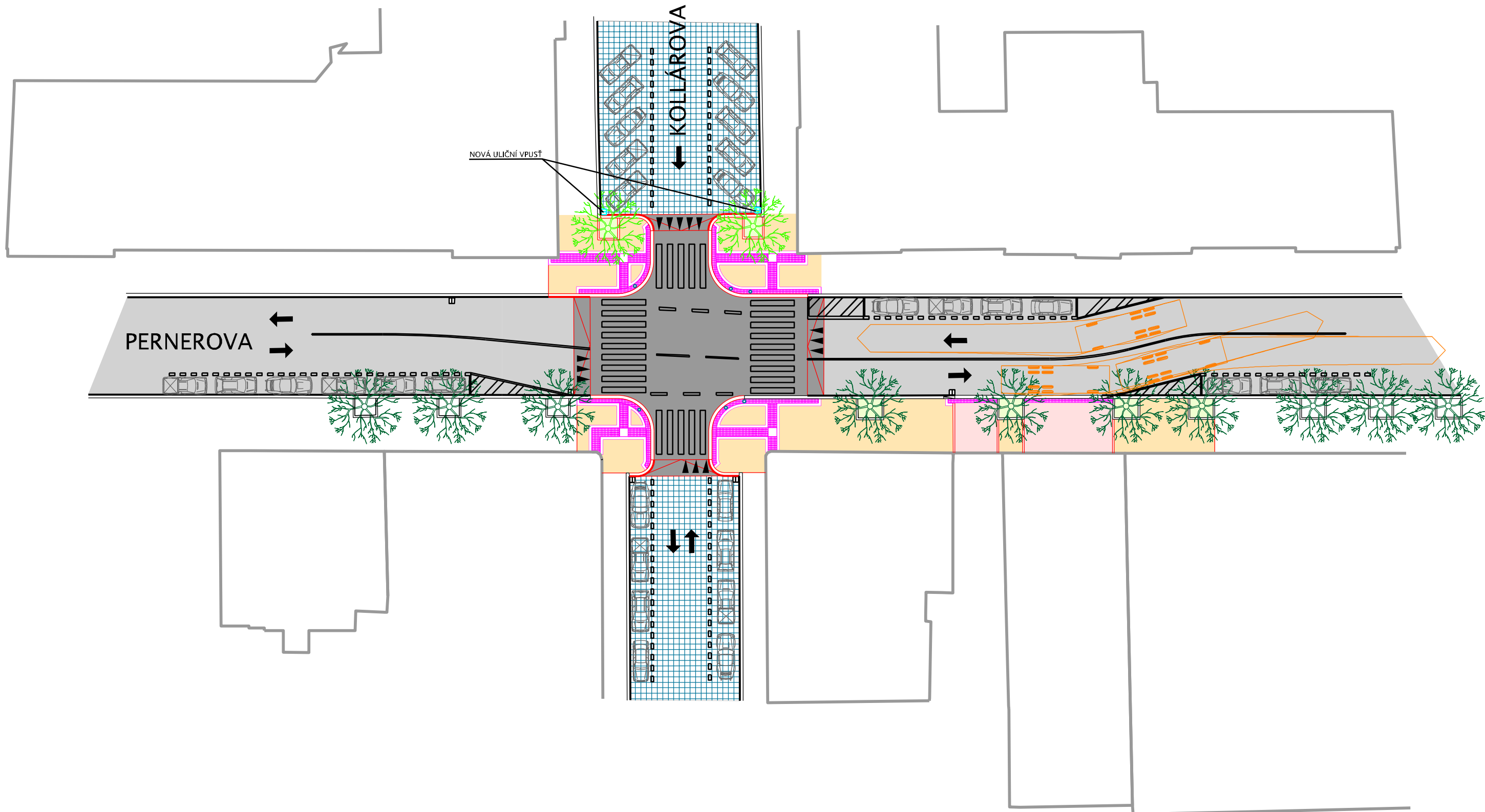
ÚPRAVA KŘIŽOVATKY PERNEROVA x KOLLÁROVA
